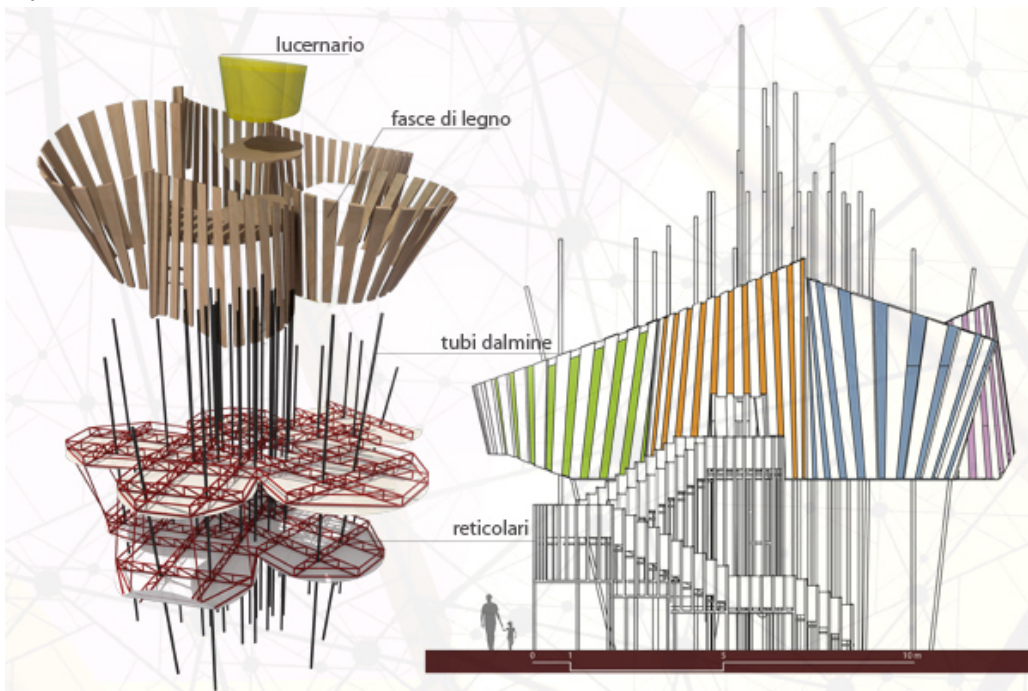
esploso e profilo
