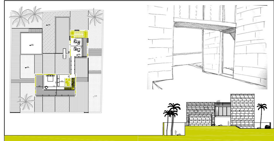
didascalia 6 pianta primo piano
