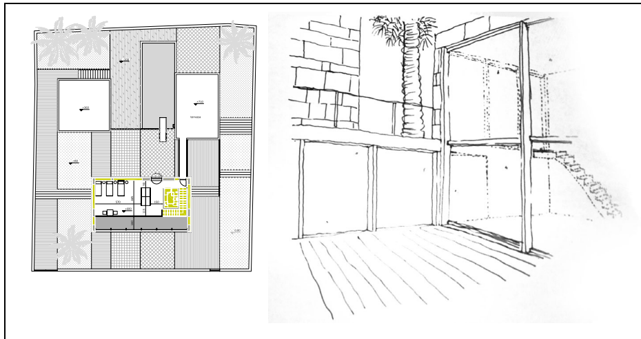
didascalia 7 pianta secondo piano
