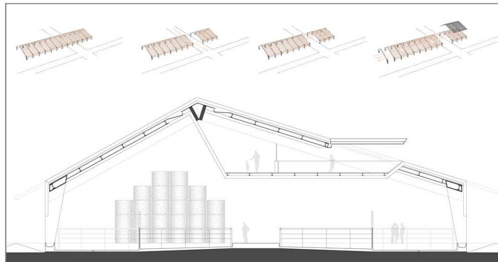
SEZIONE TRASVERSALE E SCHEMI
